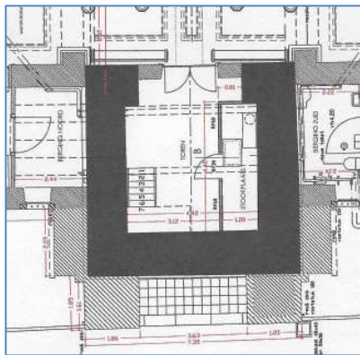
West huidige plattegrond toren Hoepertingen
